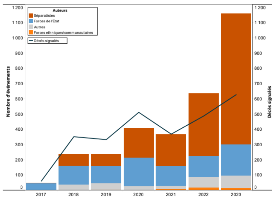
Violence ciblant les civils dans les régions anglophones par auteur, 2017-2023 168
