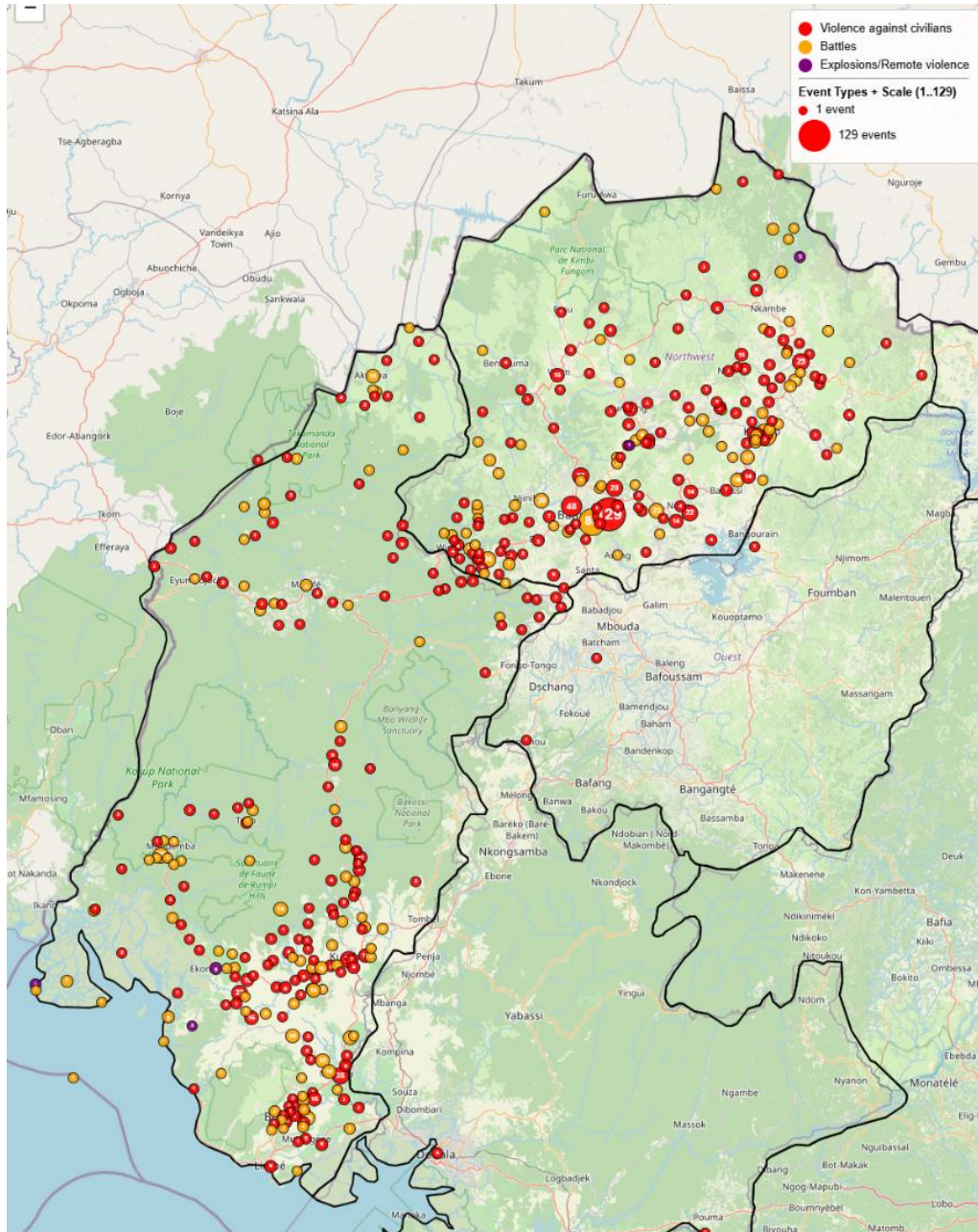
Répartition de la violence par types d'incident, 01/01/2024 – 14/03/2025. Carte réalisée par le Cedoca sur la base des données de l'ACLED 187,188
