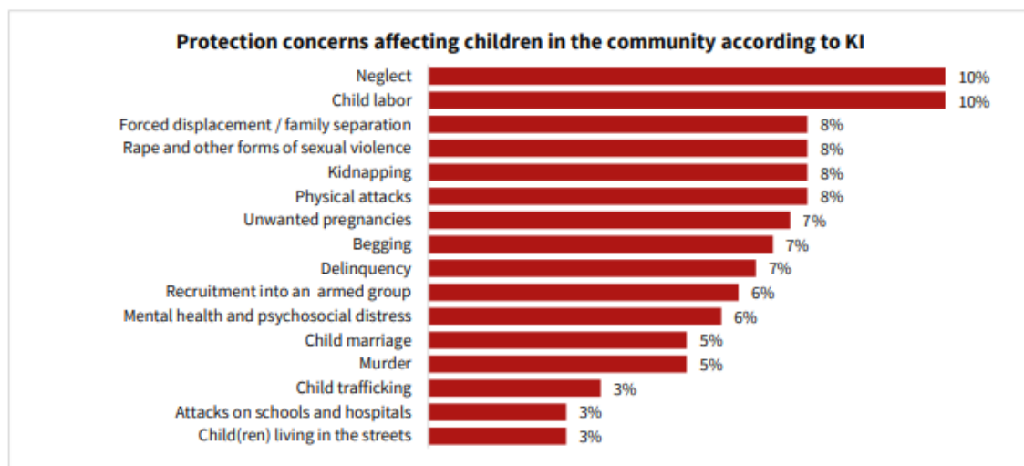
Préoccupations en matière de protection pour les enfants 224,225
