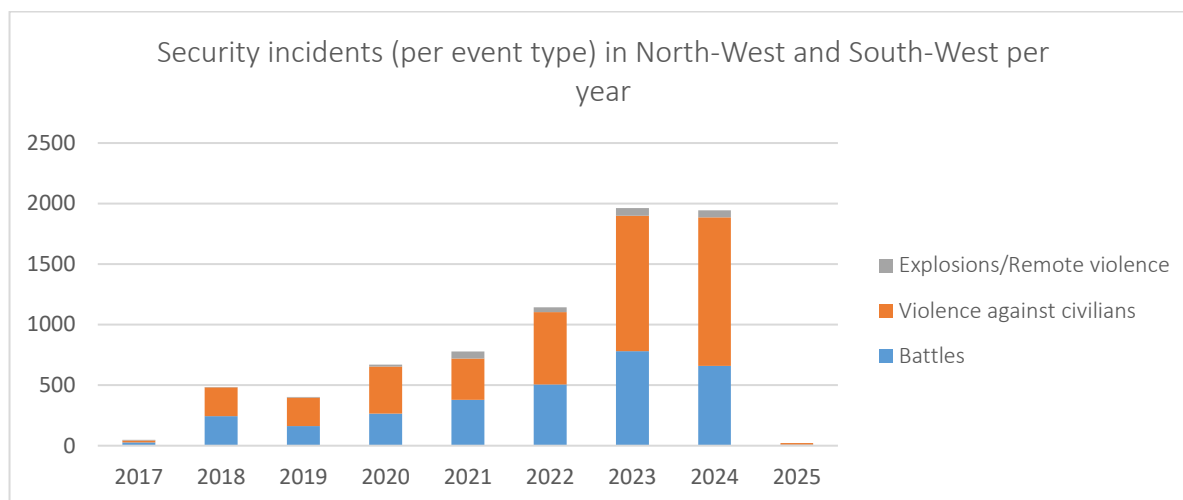
Évolution de la violence dans le NOSO par année. Graphique réalisé par le Cedoca à partir des données de l'ACLED, 01/01/2017 – 14/03/2025 95
