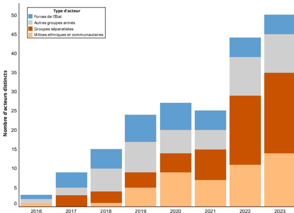
Prolifération des acteurs armés dans les régions anglophones, 2016-2023 87
