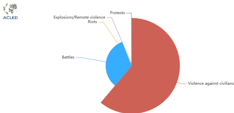
Fréquence des types d'incidents violents dans le NOSO, 01/01/2024 - 14/03/2025 172
