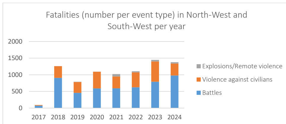
Évolution du nombre de morts par type d'incident dans le NOSO entre 2017 et 2024. Graphique réalisé par le Cedoca à partir des données de l'ACLED 156
