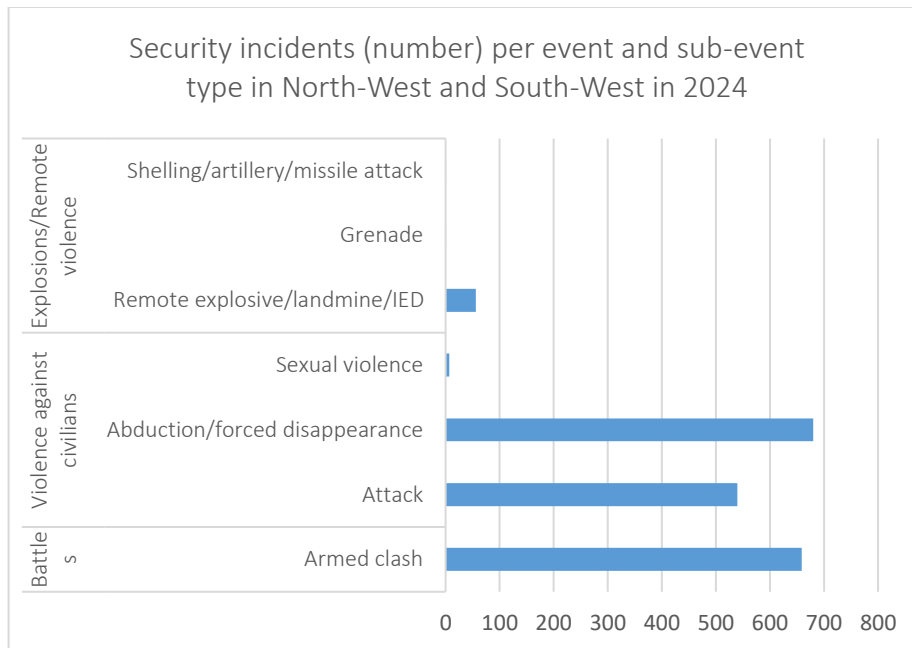
Incidents sécuritaires dans le NOSO en 2024, par types et sous-types. Graphique réalisé par le Cedoca à partir des données de l'ACLED, 01/01/2024 – 31/12/2024 93
