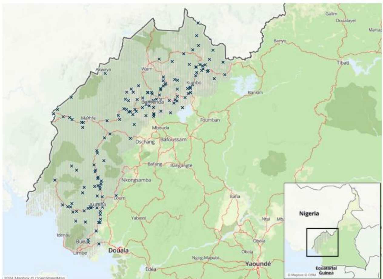
Points de contrôle dans les régions anglophones, 2017-2023 243
