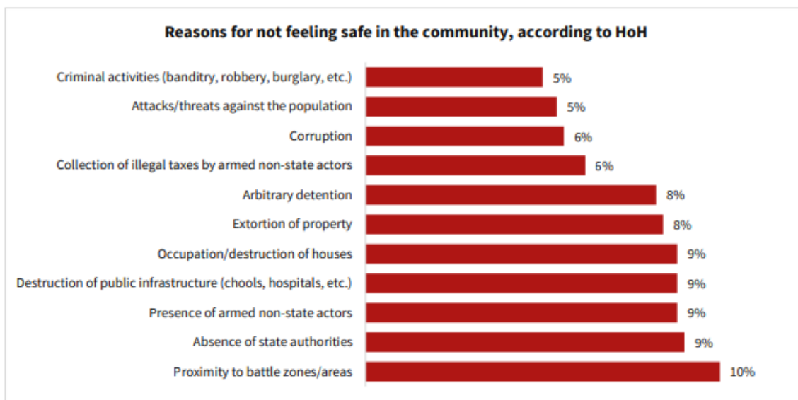
Causes principales fondant le sentiment d'insécurité 179,180
