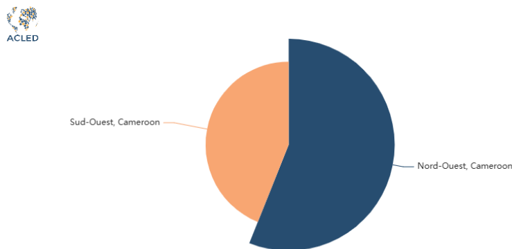
Répartition de la violence au sein des régions anglophones, 01/01/2024 – 14/03/2025 186
