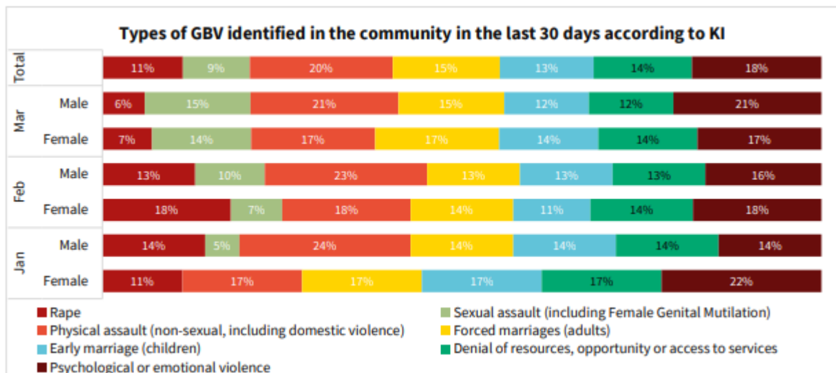
Types de VBG dans le Sud-Ouest, janvier-mars 2024 140
